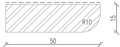
Flutterleiste L10
