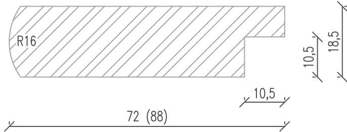
Abrollprofil L01
