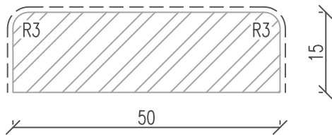
Deckleiste L03
