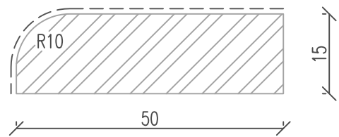
Abrolleiste L07
