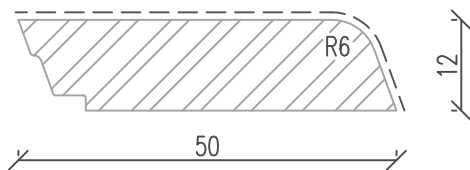
Deckleiste L21
