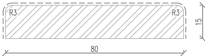
Deckleiste L04
